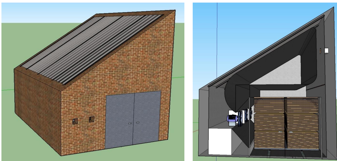
Figura 4: segundo prototipo. Vista exterior (izq.) y corte transversal (der.).
