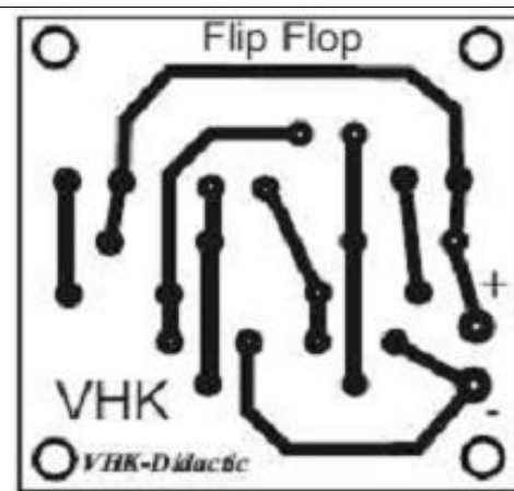
Figura N° 4 Diseño del circuito impreso
