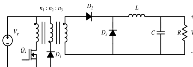
Ilustración : Convertidor Forward
