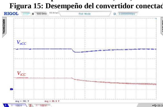
(a) Caída de la tensión de salida del boost debido a un salto de potencia no lineal de 660 W a 1,3 kW.
