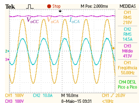
(b) Formas de ondas para carga lineal a la salida del inversor.
