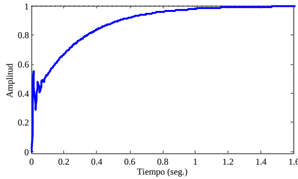
Figura 13: Respuesta al escalón unitario del sistema en lazo cerrado compensado.
