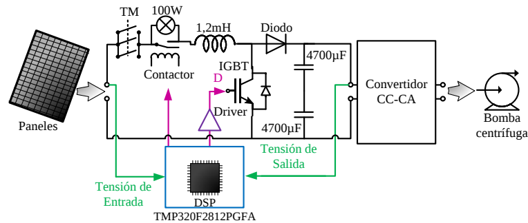
Figura 11: Esquema de un sistema fotovoltaico conectado a una bomba para riego rural.
