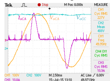
(b) Formas de ondas para carga no lineal a la salida del inversor.
