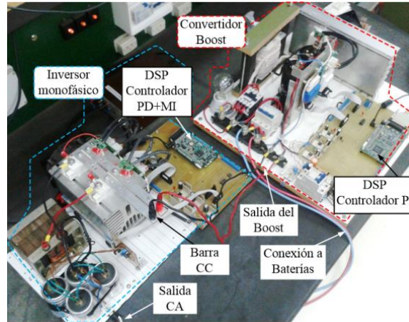
Figura 14: Fotografía del inversor (izquierda) y del boost (derecha) conectados en cascada.
