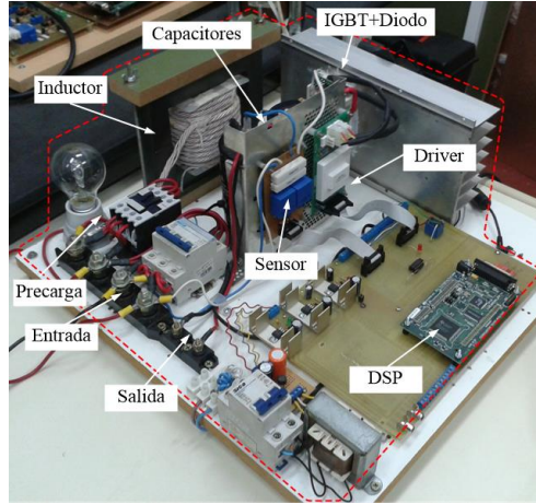
Figura 12: Prototipo del convertidor Boost montado.
